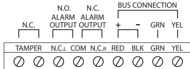
Figure 1 : Méthodes de câblage
